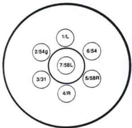
BELEGUNGSPLAN 7-POLER UNIVERSAL
