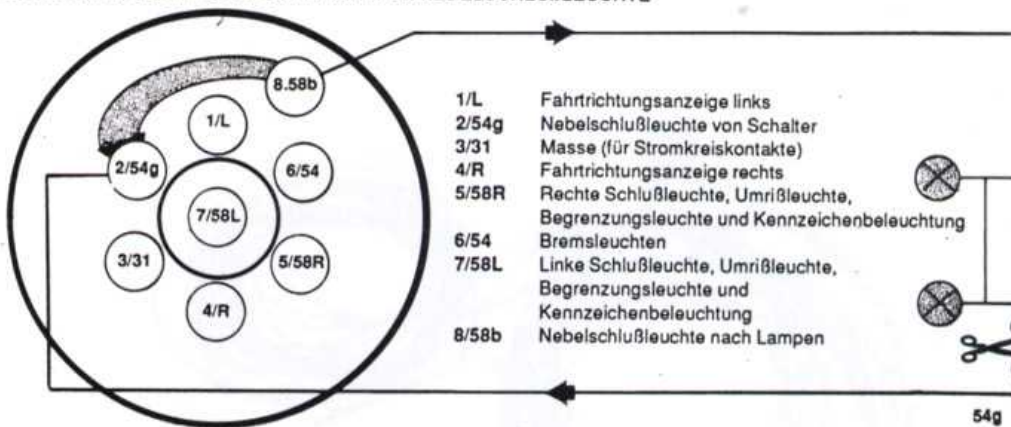
BELEGUNGSPLAN 7-POLER UNIVERSAL FÜR NEBELSCHLUßLEUCHE
