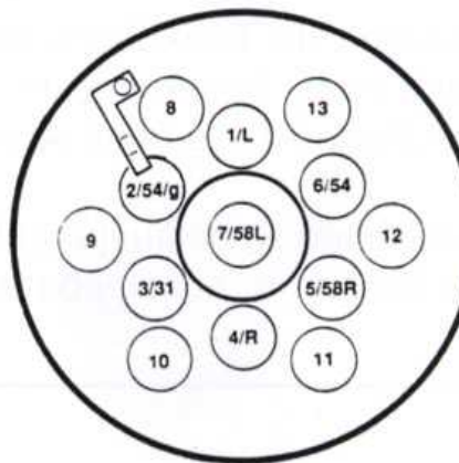
BELEGUNGSPLAN 13-POLER SYSTEM MULTICON
