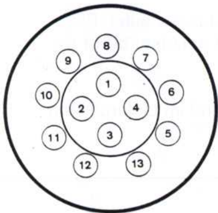
BELEGUNGSPLAN 13-POLER SYSTEM JAEGER
